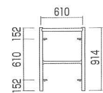
梯子型枠
