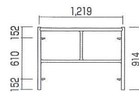
梯子型枠
