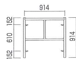
梯子型枠
