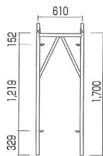
簡易型枠 (ピン付)
