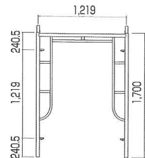
鳥居型枠 (ピン付)
