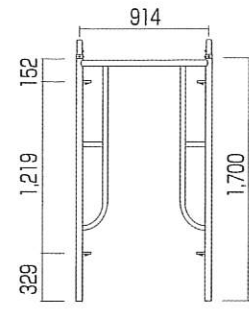
鳥居型枠 (ピン付)
