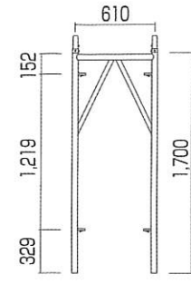
簡易型枠 (ピン付)
