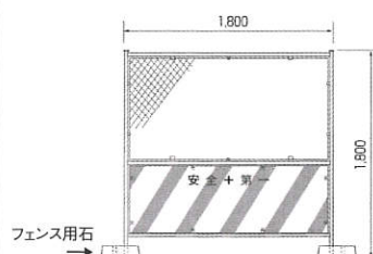
ガードフェンス・フェンス用石
