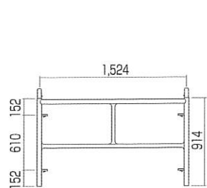
梯子型枠 (ピン付)
