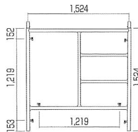
梯子型枠 (ピン付)
