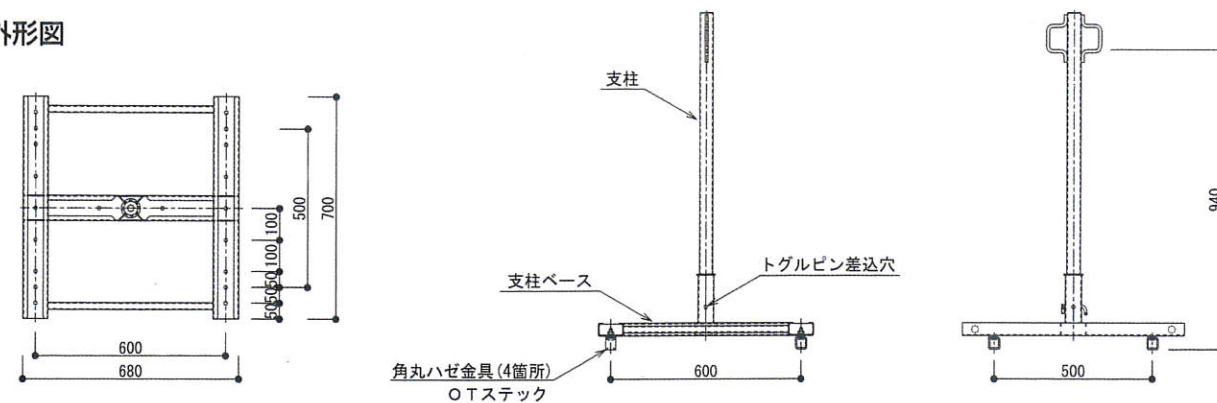
金属折板屋根墜落防護用支柱
