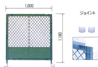
プラスチックフェンス
