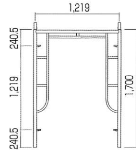
鳥居型枠 (ピン付)
