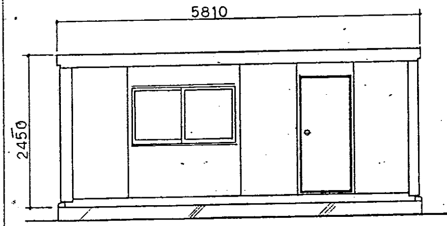
A立面図 (1/50)
