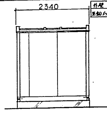
D立面図 (1/50)
