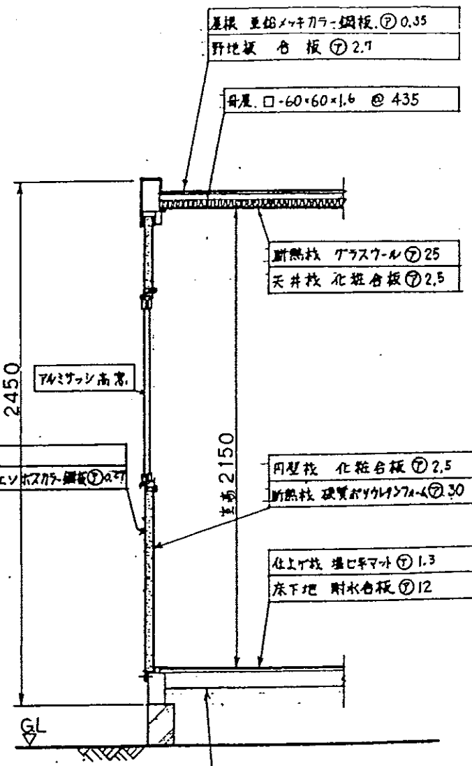
E断面矩計図 (1/20)
