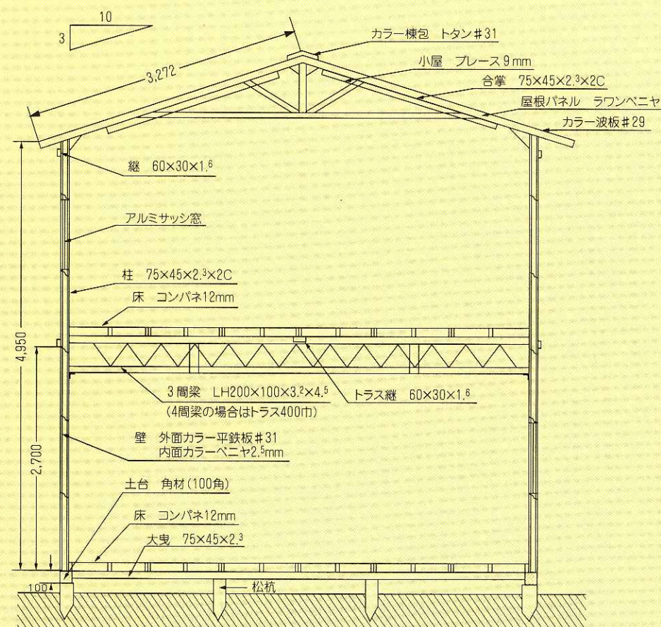
2 階建構造断面図
