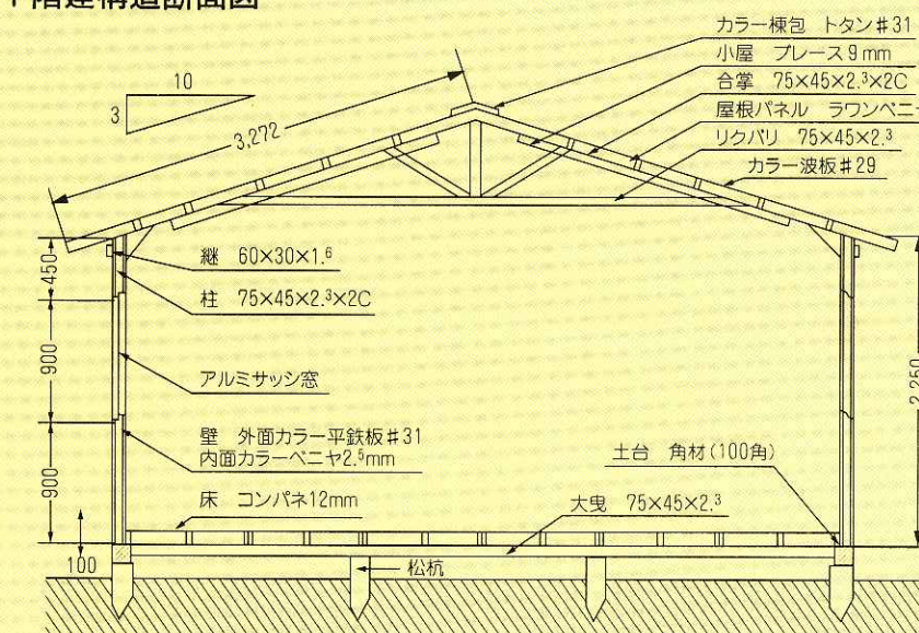
1 階建構造断面図
