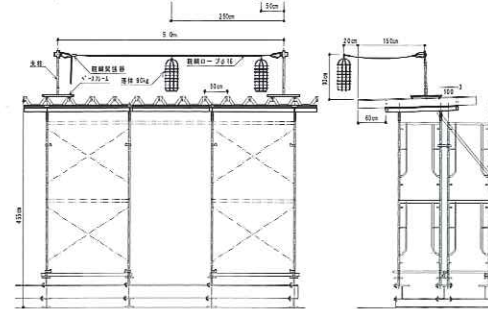
4) 墜落防護工安全基準(第2種)に基づく支柱の静荷重試験
