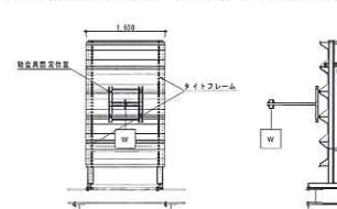
4) 墜落防護工安全基準(第2種)に基づく支柱の静荷重試験
