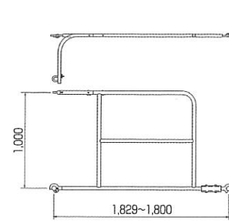
セフティガード (階段手すり枠)
