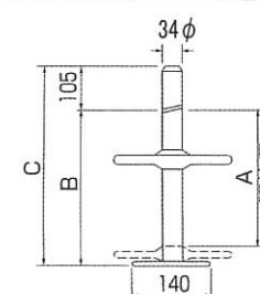
ジャッキベース
