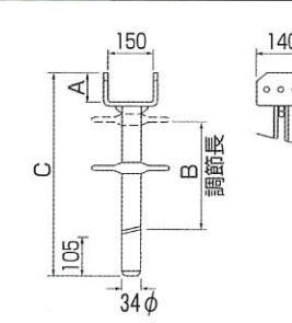
大引受ジャッキ
