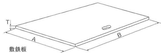
敷鉄板
