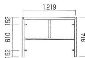
梯子型枠
